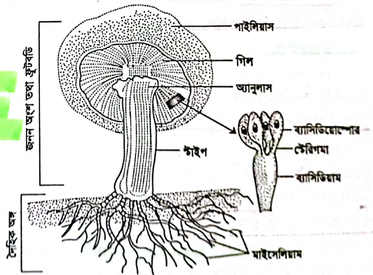
চিত্র ৫.৯ : Agaricus ছত্রাক-এর ফুটবডি এবং অন্যান্য অংশ।
