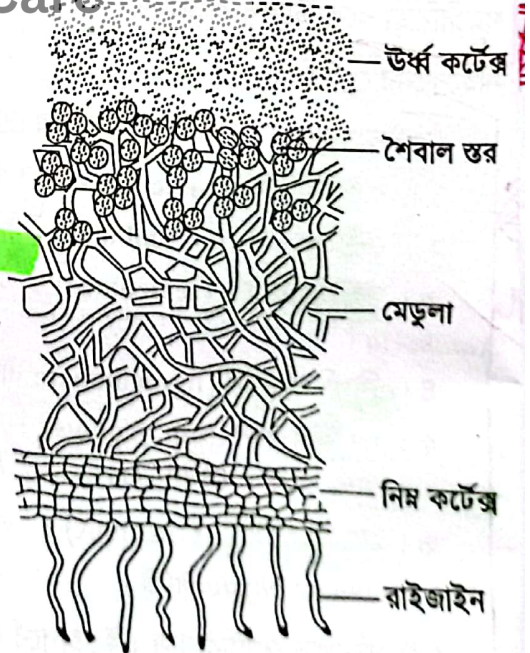
চিত্র ৫.১৪ : ফোলিয়োজ লাইকেনের অন্তর্গঠন
